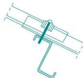
FIXATION EN SOMMET D'ONDE
