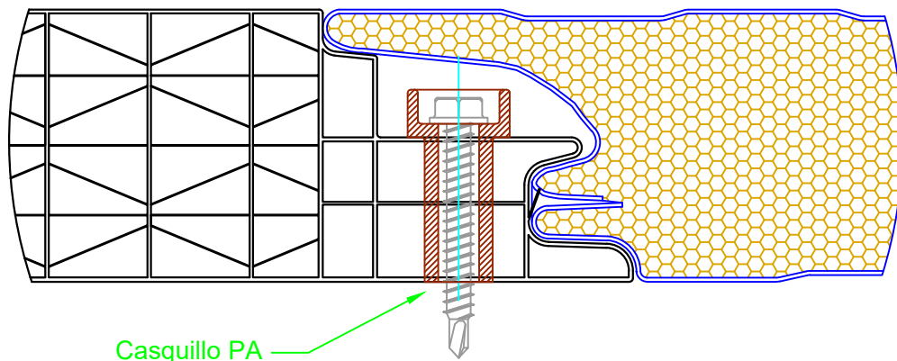
DETALLE ENCUENTRO CON METECNO Superwall 40 ESCALA 1:1
