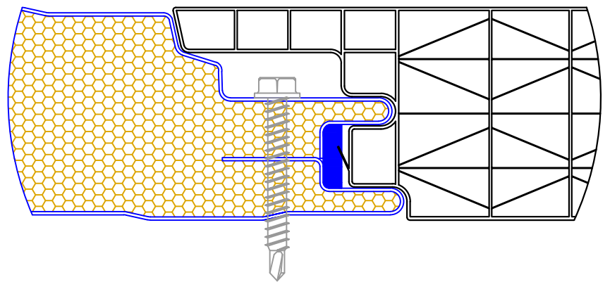
DETALLE ENCUENTRO CON METECNO Superwall 40 ESCALA 1:1
