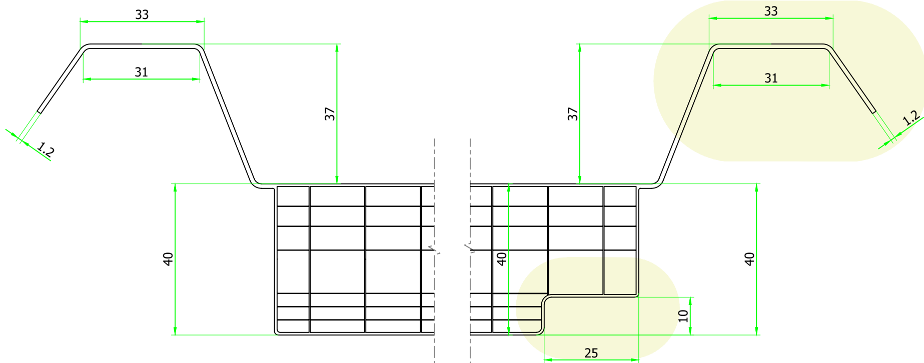
DETALLE LADO A ESCALA 1:1
